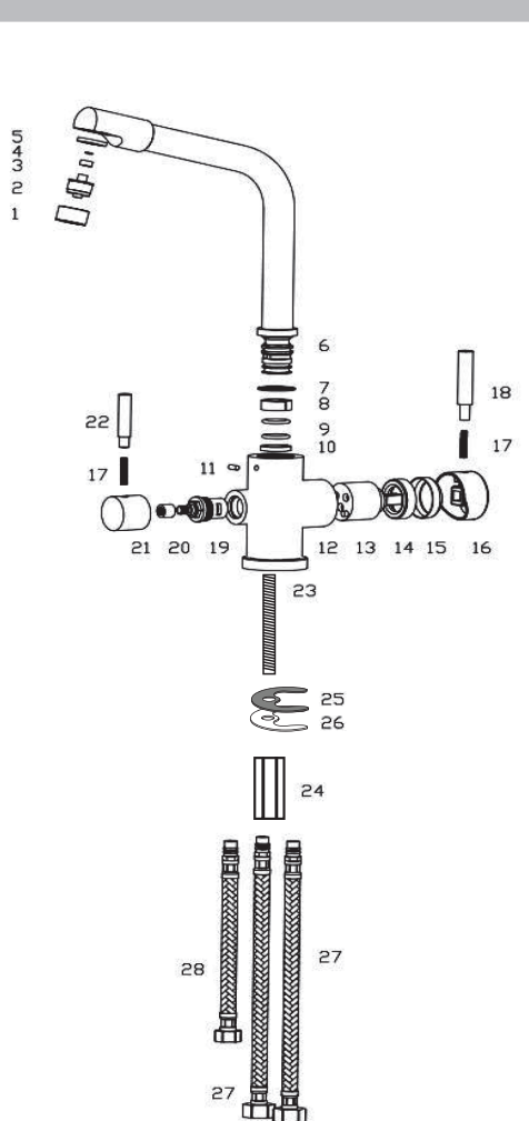
Рис. 1. Детали смесителя
