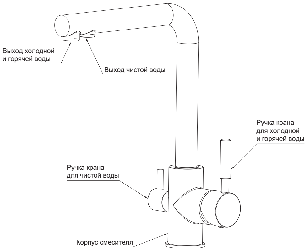
Рис. 3. Смеситель в сборе
