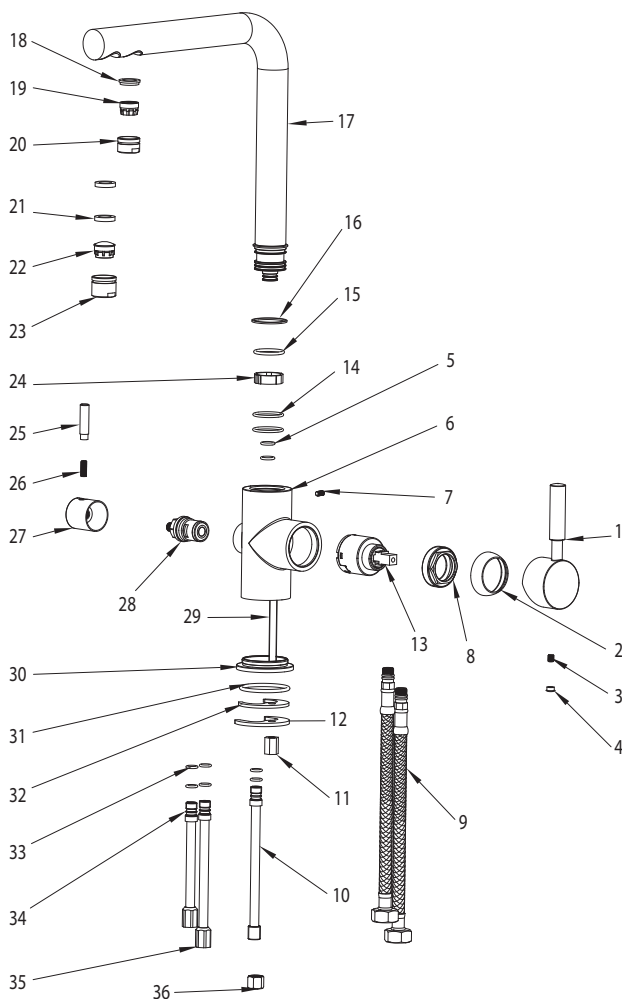
Рис. 1. Детали смесителя
