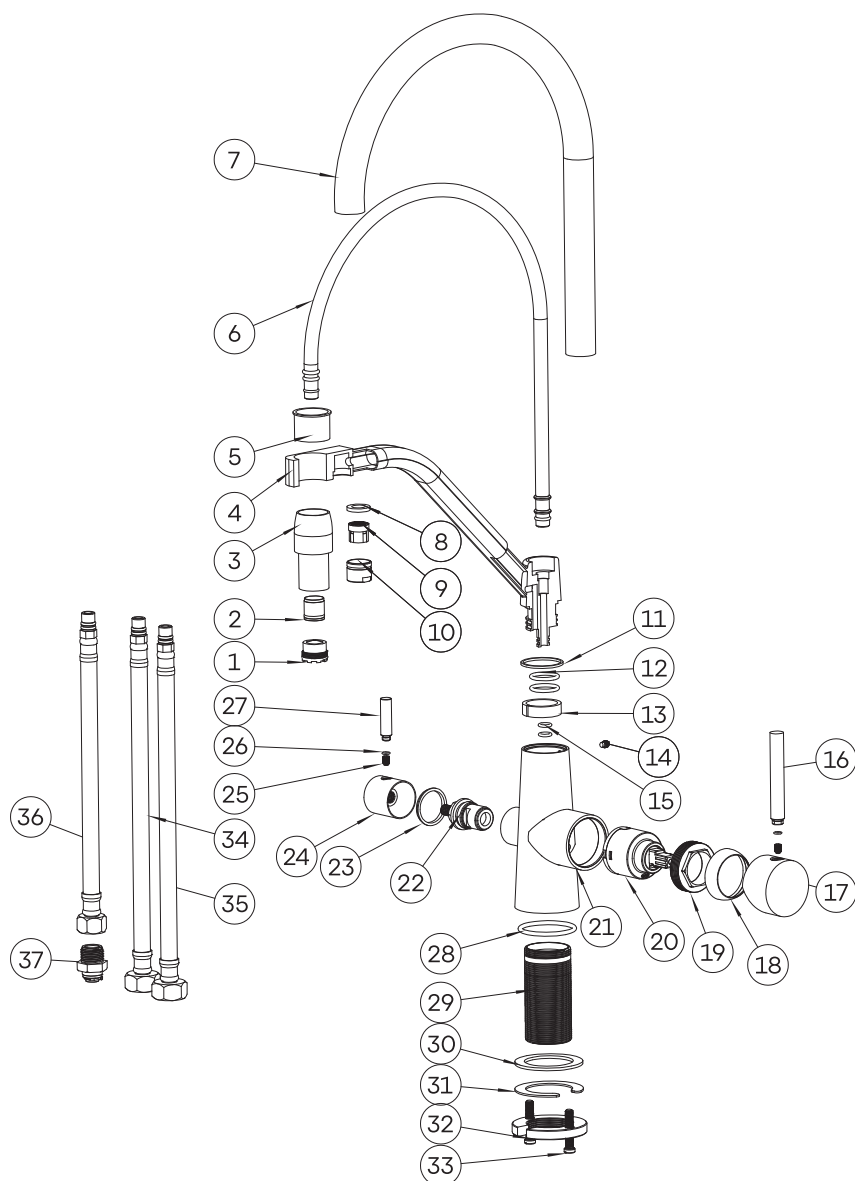
Рисунок 1. Составляющие компоненты смесителя
